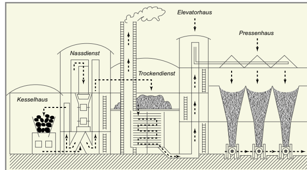
Funktionsschema einer Brikettfabrik
